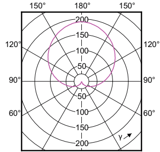
(cd/1000lm) 0° 150° 180° 150°
