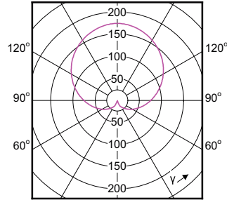
(cd/1000lm) 0° 150° 180° 150°
