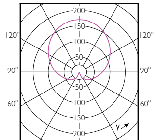
(cd/1000lm) 0°
