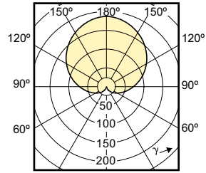
(cd/1000lm) 0° 150° 180° 150°
