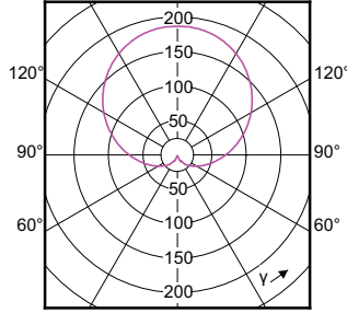
(cd/1000lm) 0° 180° 150°
