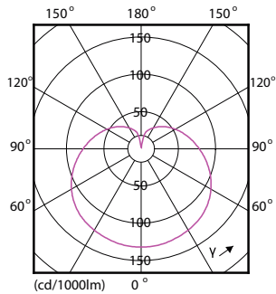
CorePro LEDlustre 40W E14 865 FR P45
