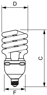
HL HS HV 10Kh EMI HPF 45W 220-240V E27WW
